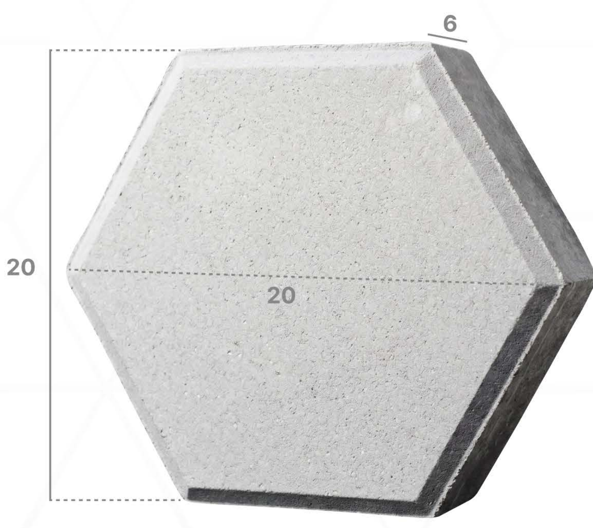
SEGI ENAM 6 CM
