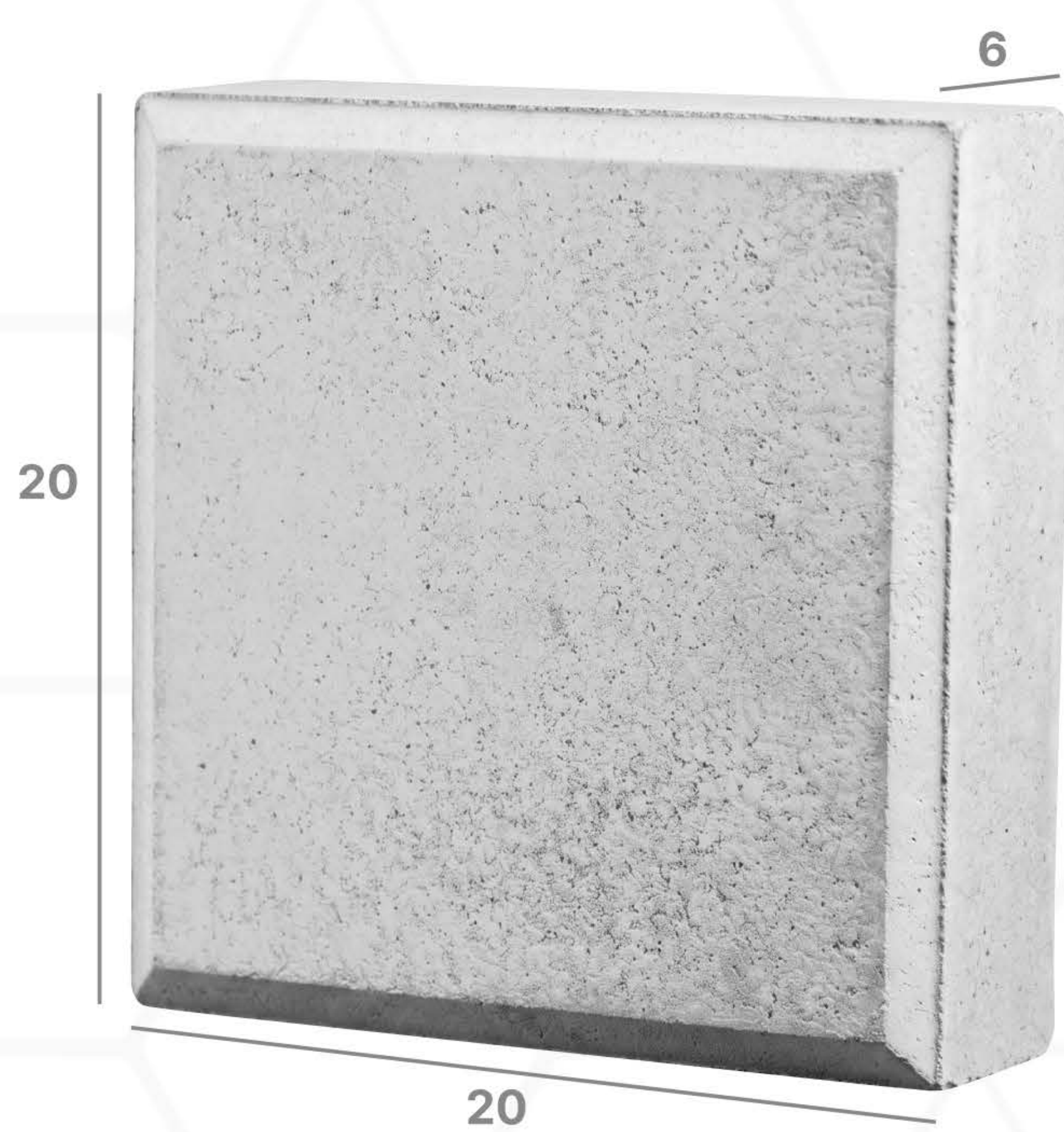
BUJUR SANGKAR 6 CM
