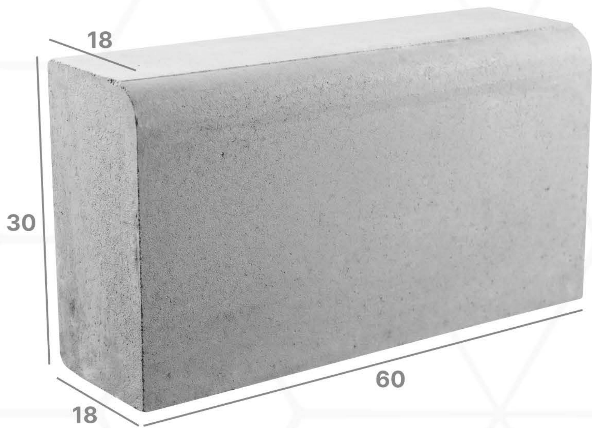
PAVING KANSTIN TROTOAR
